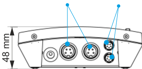
Ansicht Anschlüsse
